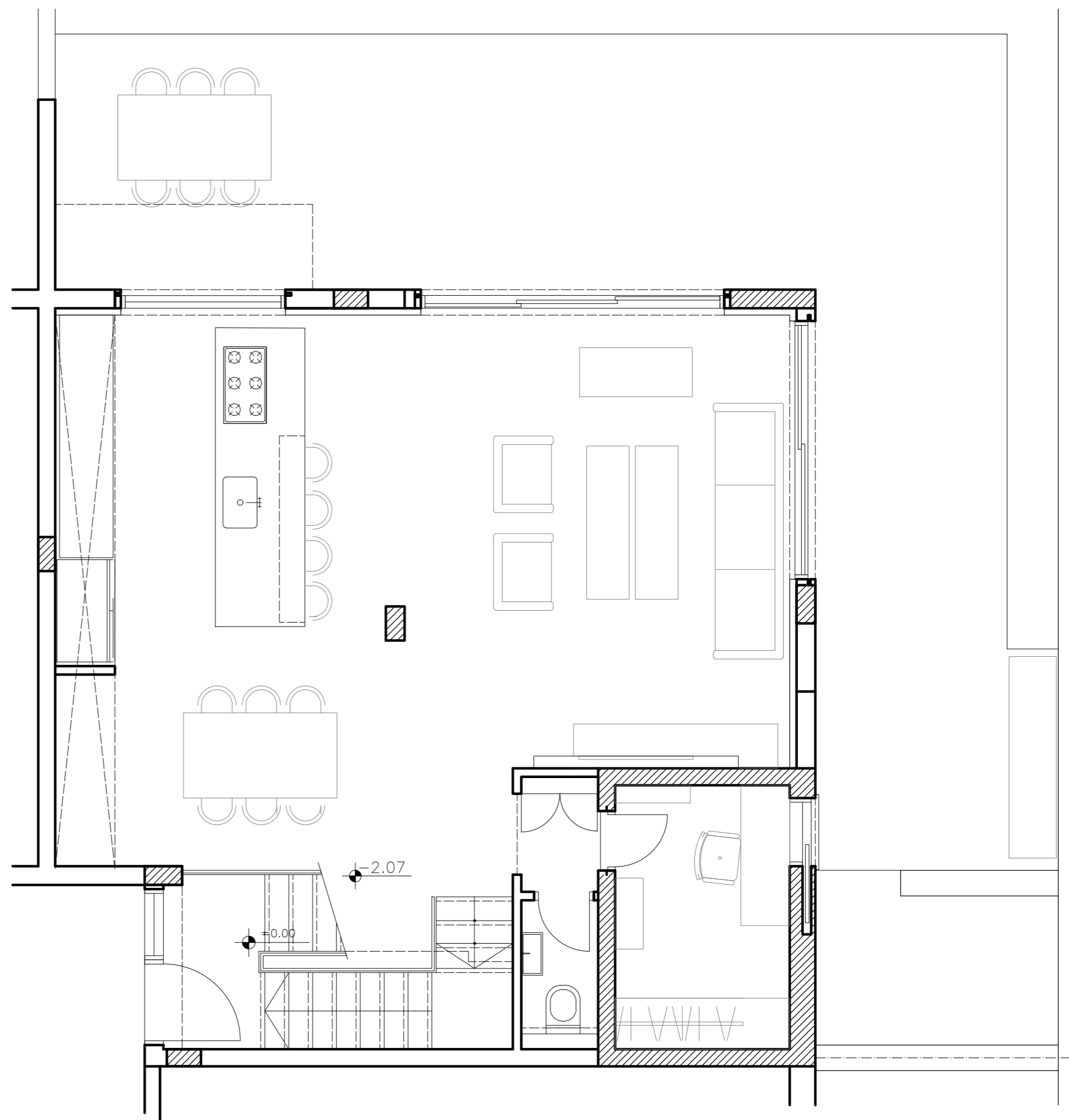
קומת קרקע
